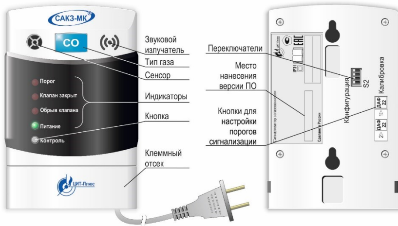
Рисунок 1 – Внешний вид сигнализаторов
