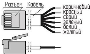
Вилка на кабель ТP6P6C Розетка G2U3000-SK-1G Рисунок В.3 – Схема подключения клапана КЗЭУГ с разъемом ТJ1А-6Р6С
