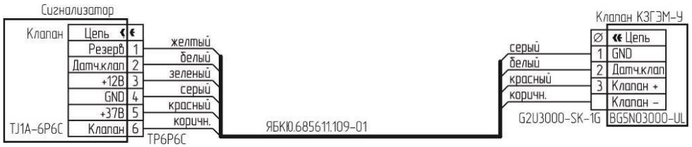
Рисунок В.1 – Схема подключения КЗГЭМ-У с разъемом ВG5N03000-UL
