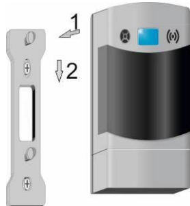
Рисунок 3 – Установка сигнализатора
